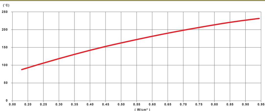
Variatione della temperatura superficiale di un riscaldatore in silicone di 2.5mm di spessore in funzione del carico di potenza superficiale. Il riscaldatore è sospeso in aria calma, non fissato su una superficie metallica, ad una temperatura ambiente di 25^{\circ}C . Il riscaldatore non è protetto da un sistema di limitazione della temperatura. In queste condizioni, il riscaldatore si danneggia irreversibilmente a 235^{\circ}C .
